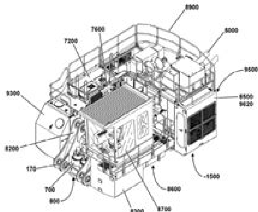
Fig. 1.1.2 Uppercarriage
