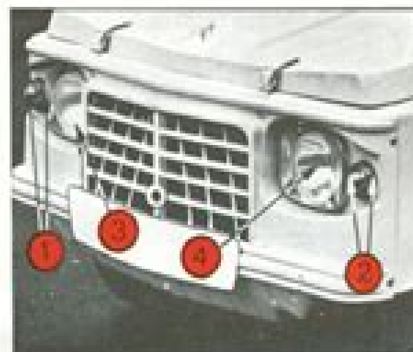
Fig. 46 - Luces de señalización delanteras 1-2 - Indicadores de dirección 3-4 - Luces de posición con las parábolas de los faros
