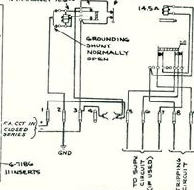
SCHEMATIC WIRING
