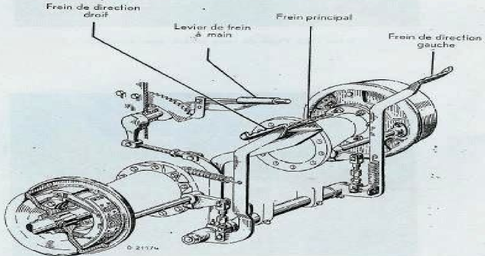
Grav. 179: Freins des roues arrière
