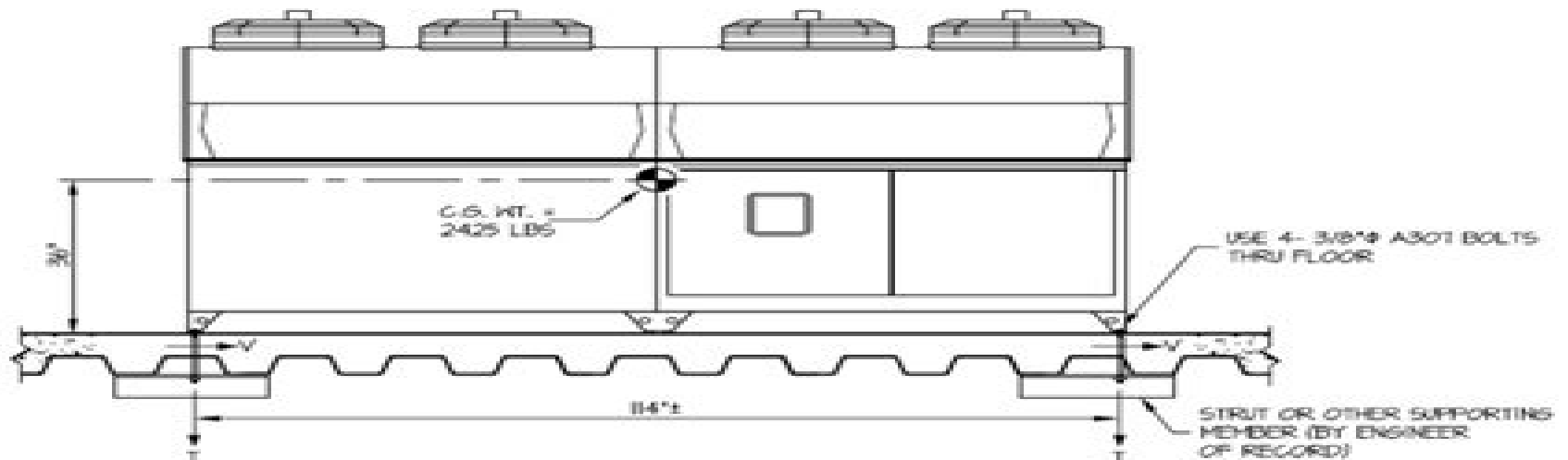
ELEVATION
