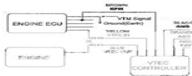
VTEC CONTROLLER WIRES
