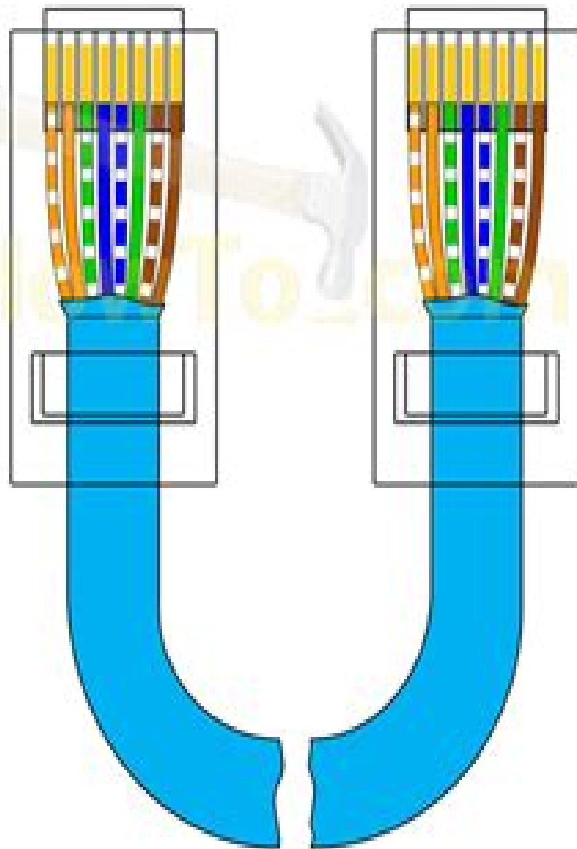
EIA/TIA T568B
