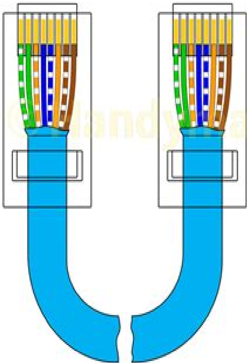
EIA/TIA T568A
