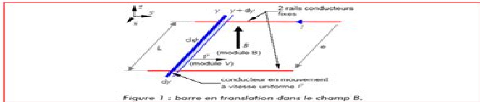
Figure 1 : barre en translation dans le champ B .
