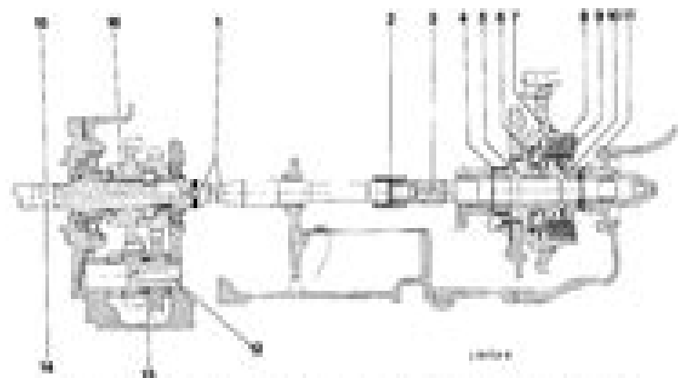
Bild 2 - Verschiebbare, kombinierte Zapfenwelle für 540 U/min und 1000 U/min - Schnitt
