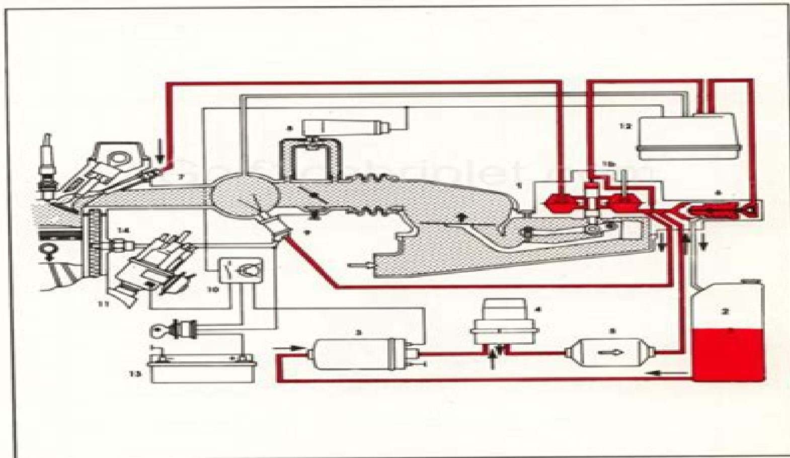
Figure 1 - Schéma du système K-Jetronic
