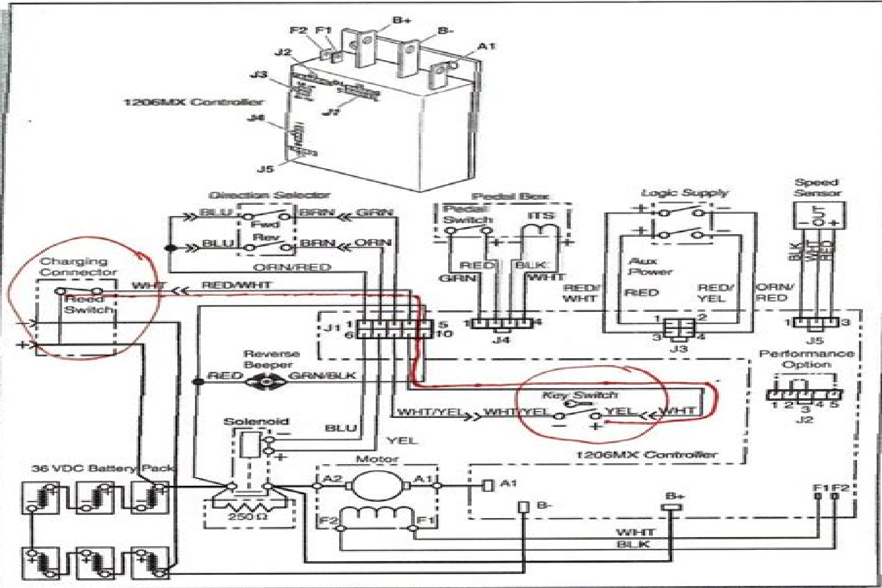
Fig. 9 Wiring Diagram
