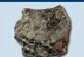
28. Sphalerite
