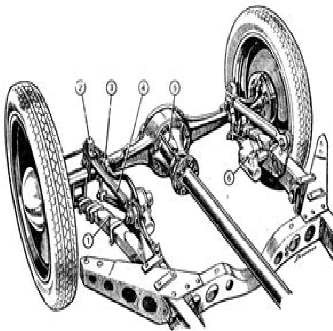
Fig. 12.37. Achtereinde van een oude Fiat 500, met kwartelliptische veer. 1. kwartelliptische veer; 2. bevestiging schokbrekerarmen en reactiestaven; 3. remolieleidingen; 4. reactiestaven; 5. differentieelhuis; 6. schokbrekers.
