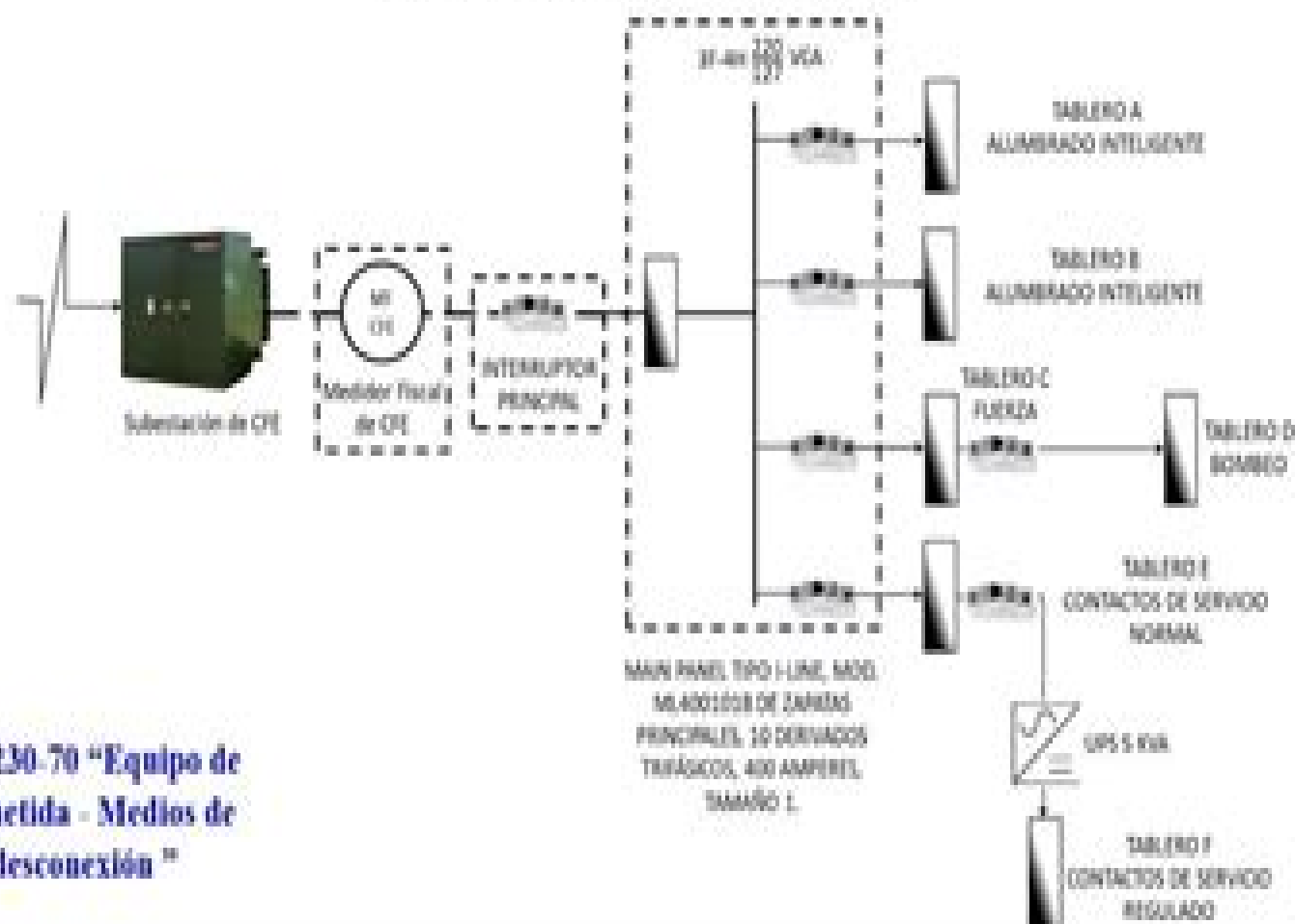
Diagrama Unifilar del Sistema de Distribución Secundaria
