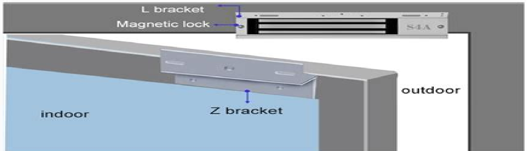
Single door display diagram
