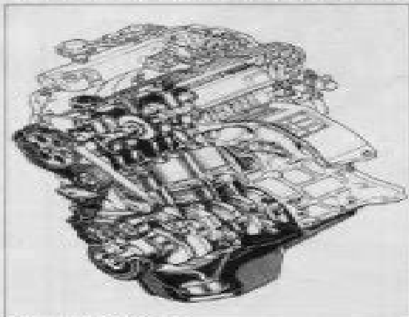
Двигатель 3S-FE, 4S-FE
