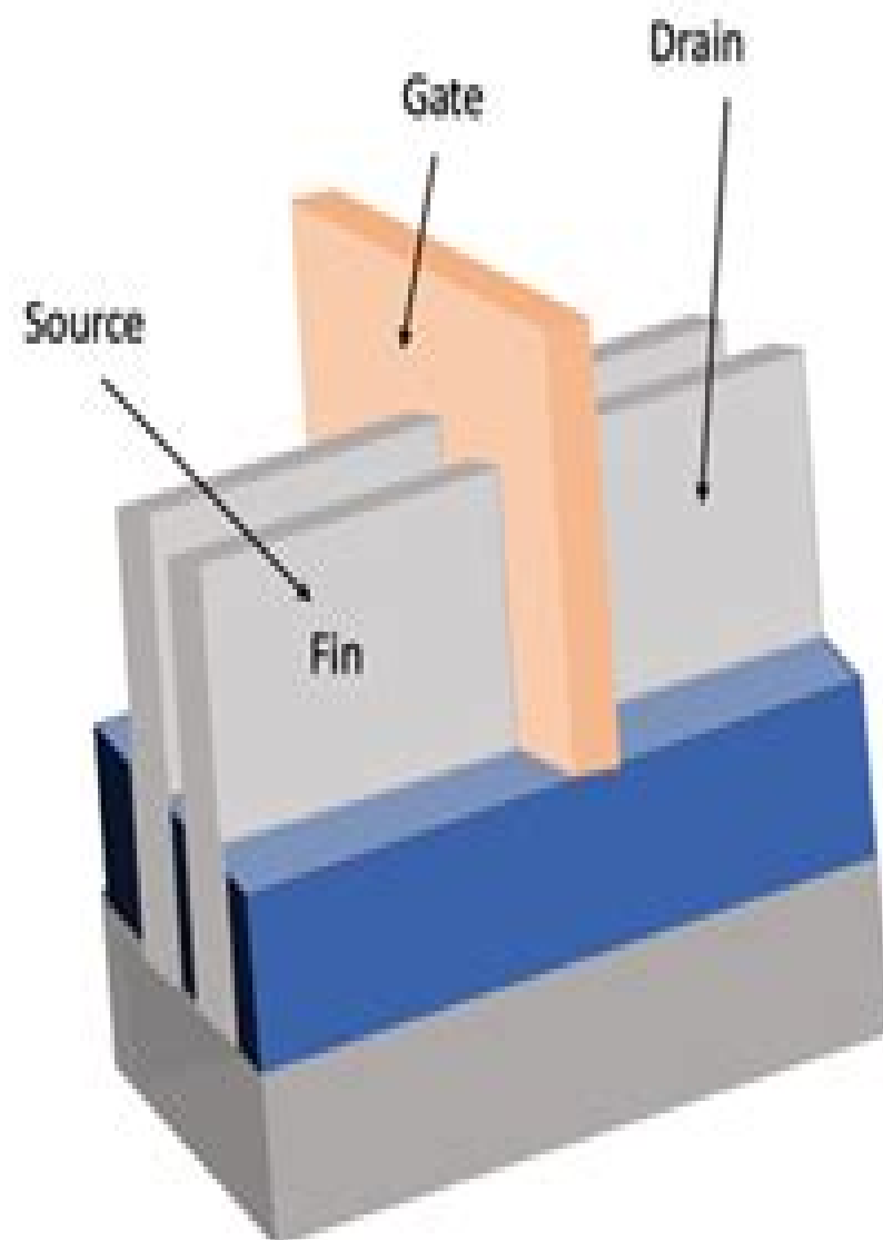
3-D FinFET
