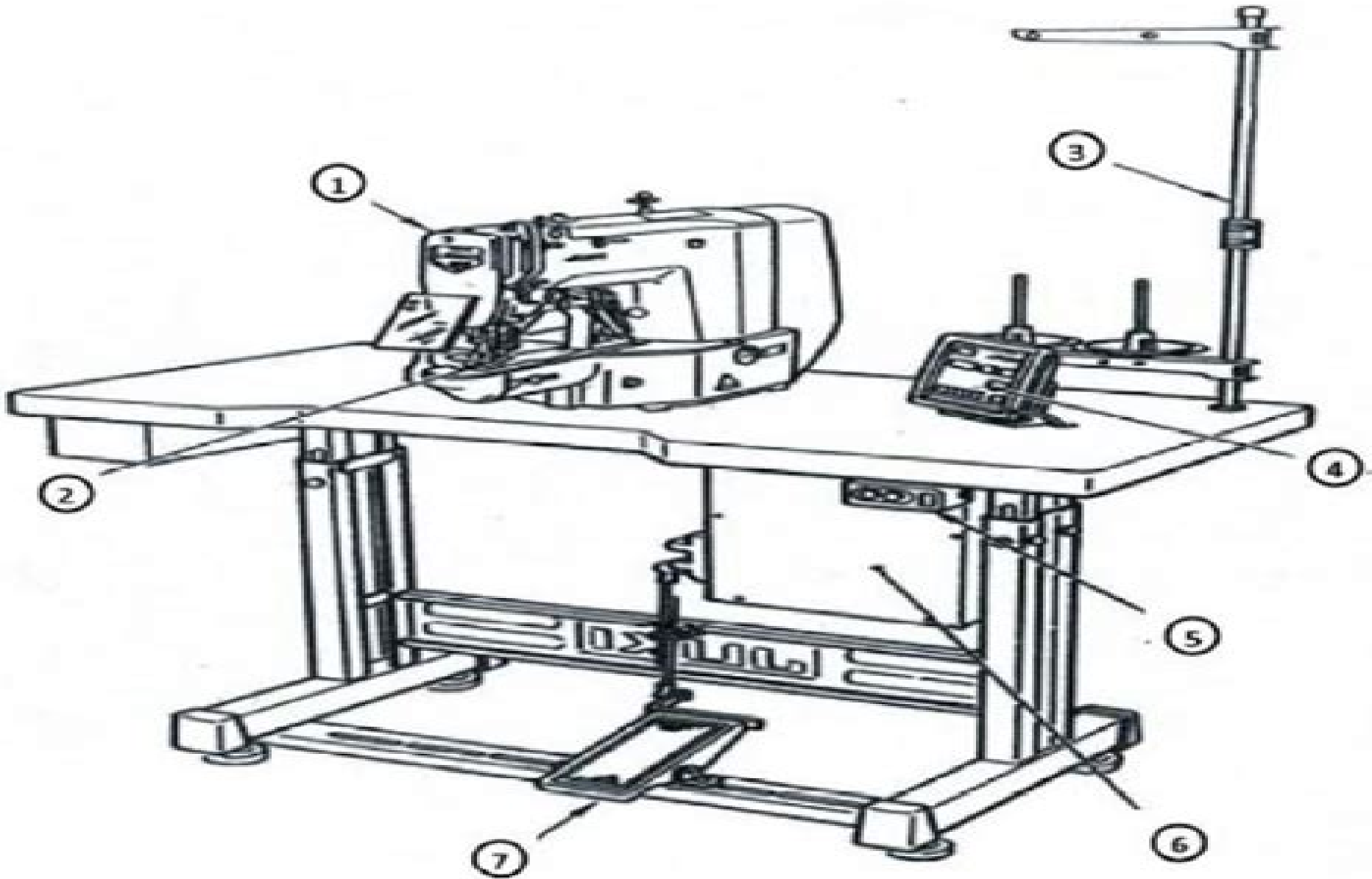
Máy đính bọ LK1900A-SS và đính cúc LK1903A-SS 1-Đầu máy; 2-Bàn kẹp; 3-Già chỉ; 4-Bảng điều khiển; 5-Công tắc nguồn; 6-Hộp điện tử; 7-Bàn đạp.
