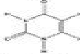
Uracil
