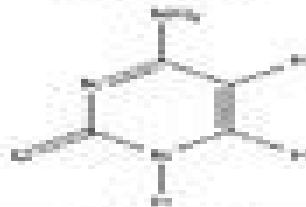
Cytosine
