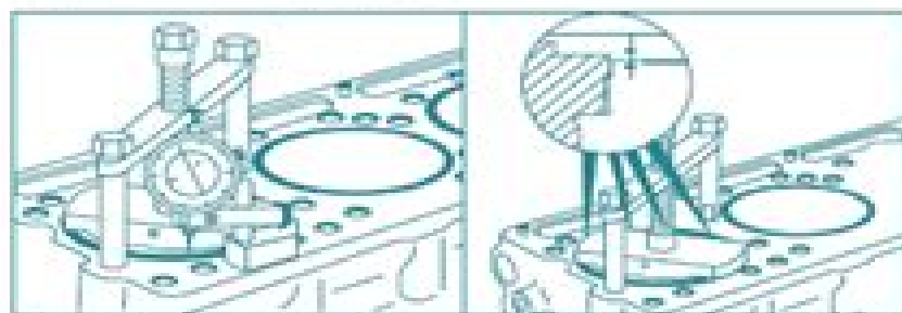
Dimensiones de las camisas de cilindros Navistar 360 - 466
