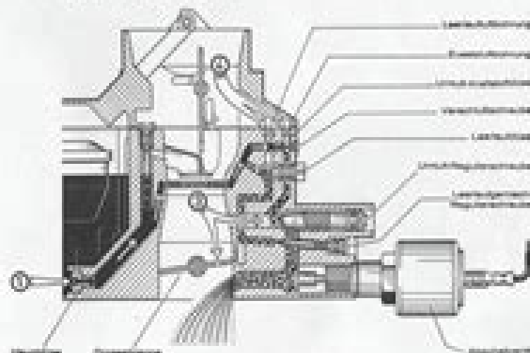
Bild 10: 34 PICT-3 Wirkungsweise des Leerlauf- und Umluftsystems ① = Zufuhr des Kraftstoffes ② = Eintritt der Ausgleichluft ③ = Eintritt der Leerlaufluft
