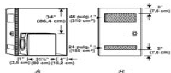
A. Vista lateral - clóset o lugar confinado B. Puerta de clóset con orificios de ventilación
