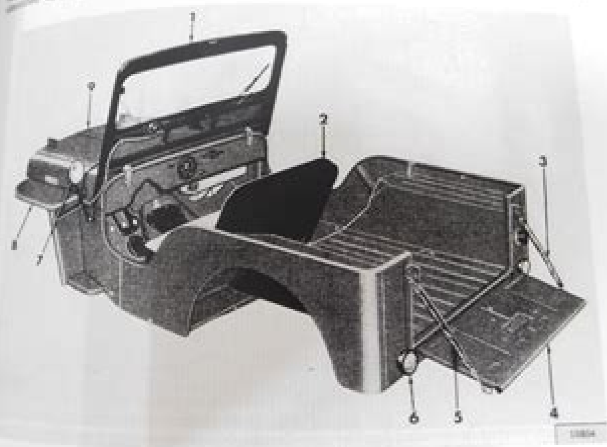
FIG. 341—MODEL DJ-3A BODY
