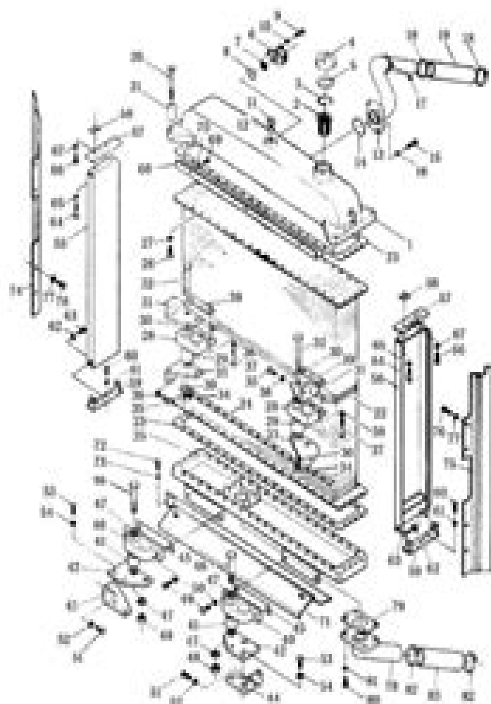
第106图 散热器 FIG106 RADIATOR
