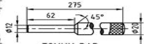
TOMMY BAR (MILD STEEL)
