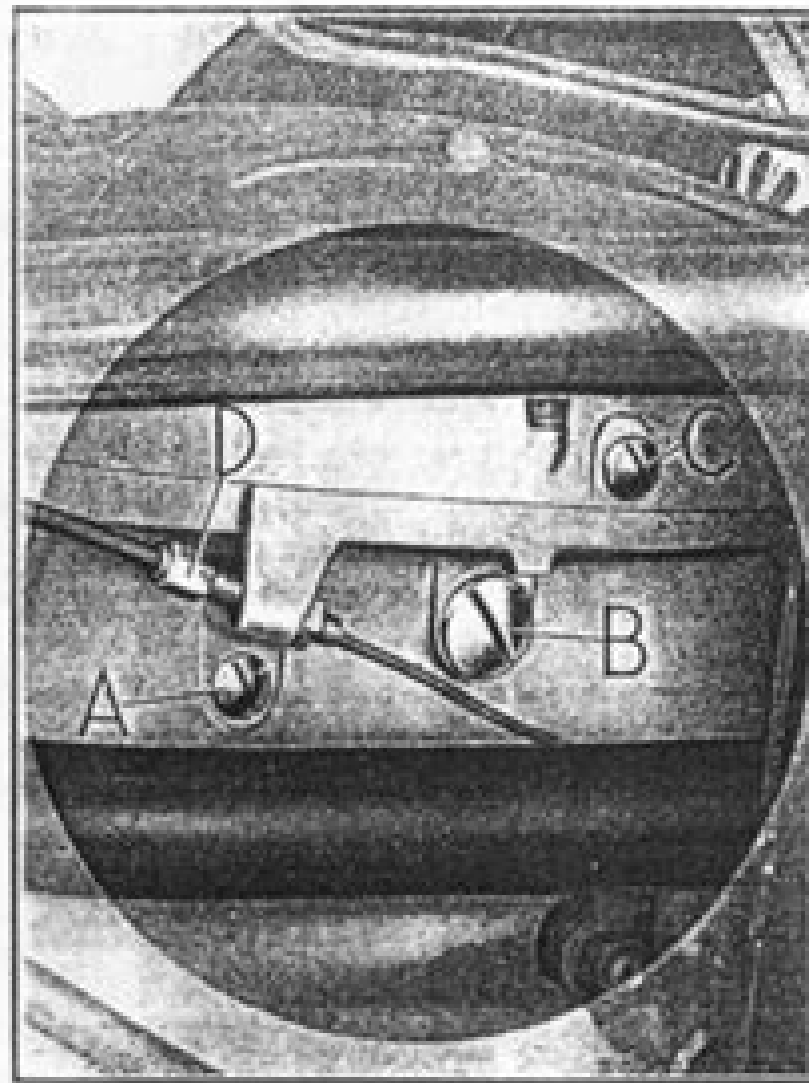
Obr. 12. Výpustné šrouby oleje a stavěcí šroub bowdenu spojky
