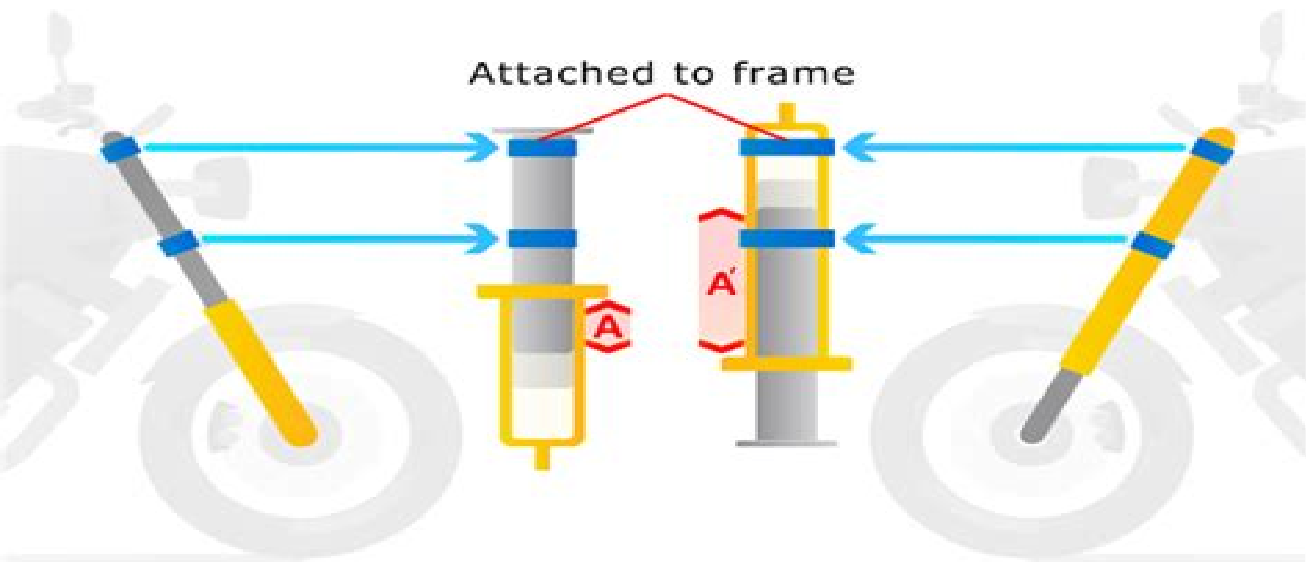
Upright Forks
