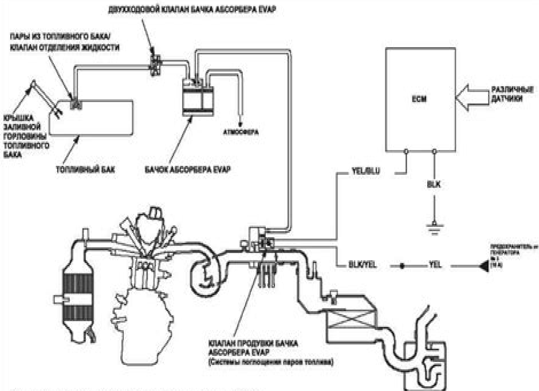
Схема системы управления абсорбером паров топлива (EVAP)
