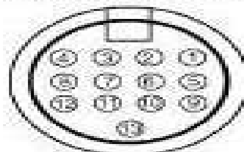
<CN703 13P CONNECTOR>
