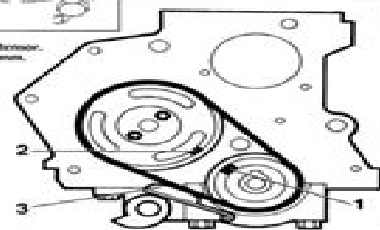
Calado de la distribución.
