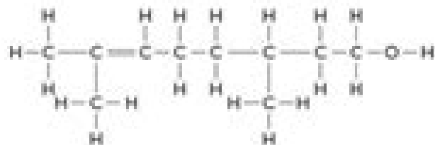
citronellol
