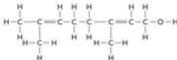
geraniol
