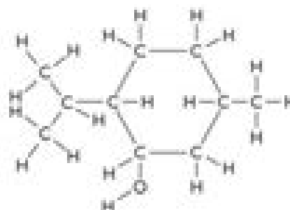
menthol
