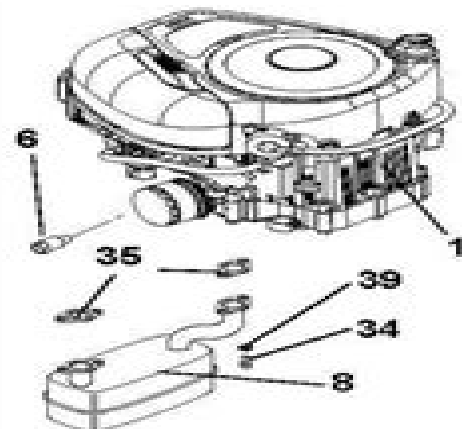
Muffler: 915213, 215
