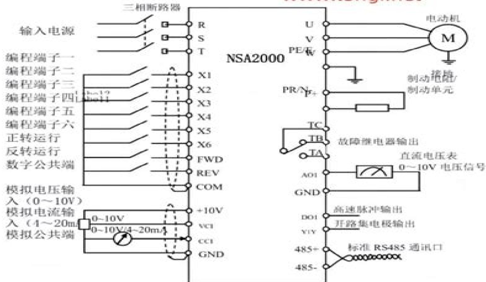
基本配线图
