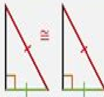
RHL Right-Hypotenuse-Leg
