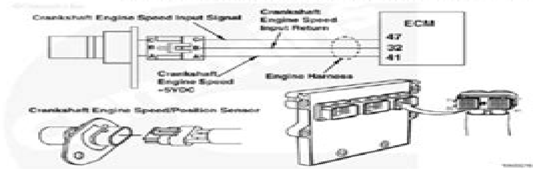
Circuito del Sensor de Velocidad/Posición del Cigüeñal del Motor
