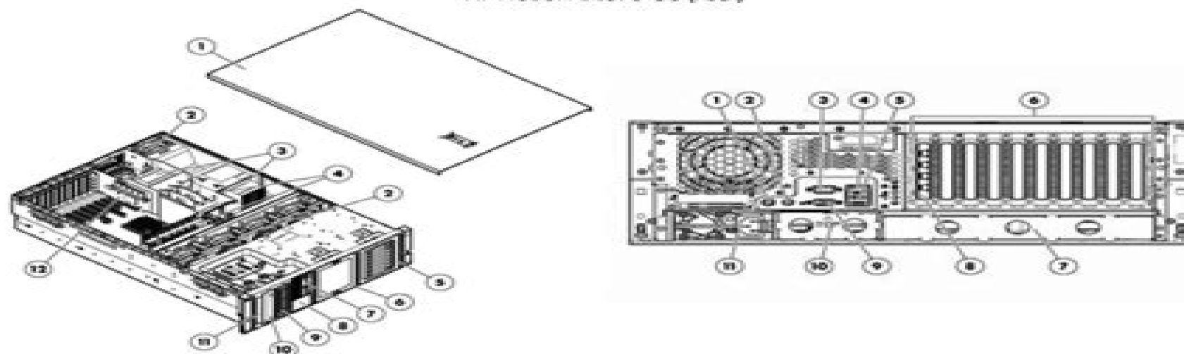
HP ProLiant DL370 G6 (Rock)
