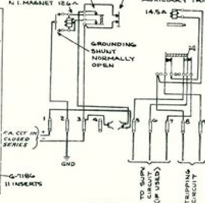
SCHEMATIC WIRING
