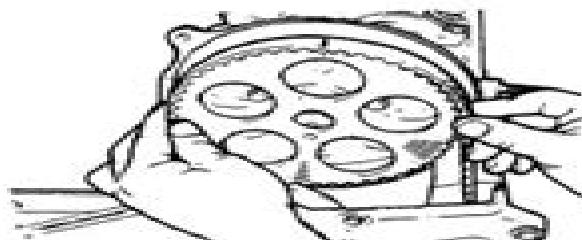
Installing camshaft sprocket (4G33)
