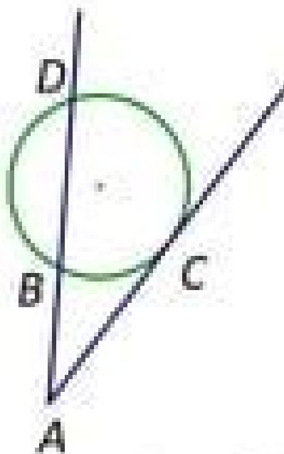
Secant-Tangent
