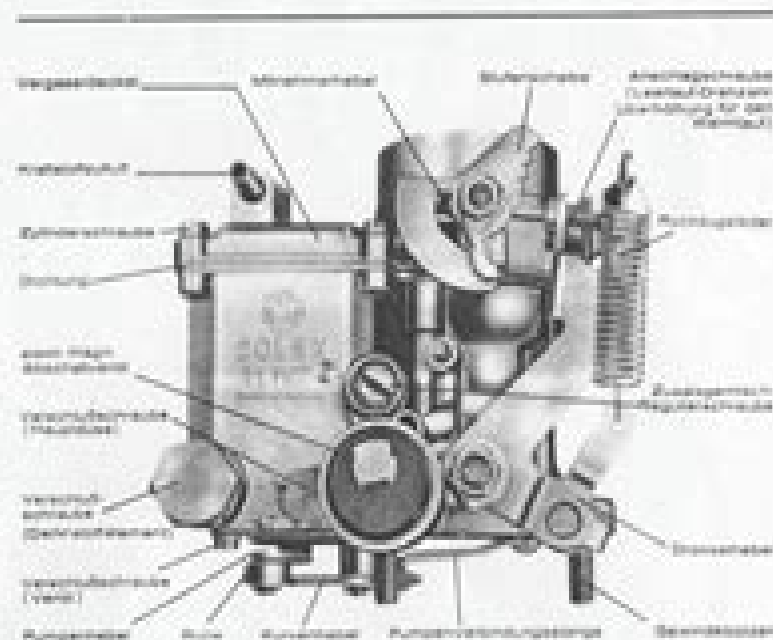
Bild 17: SOLEX-Fallstromvergaser 31 PICT-4
