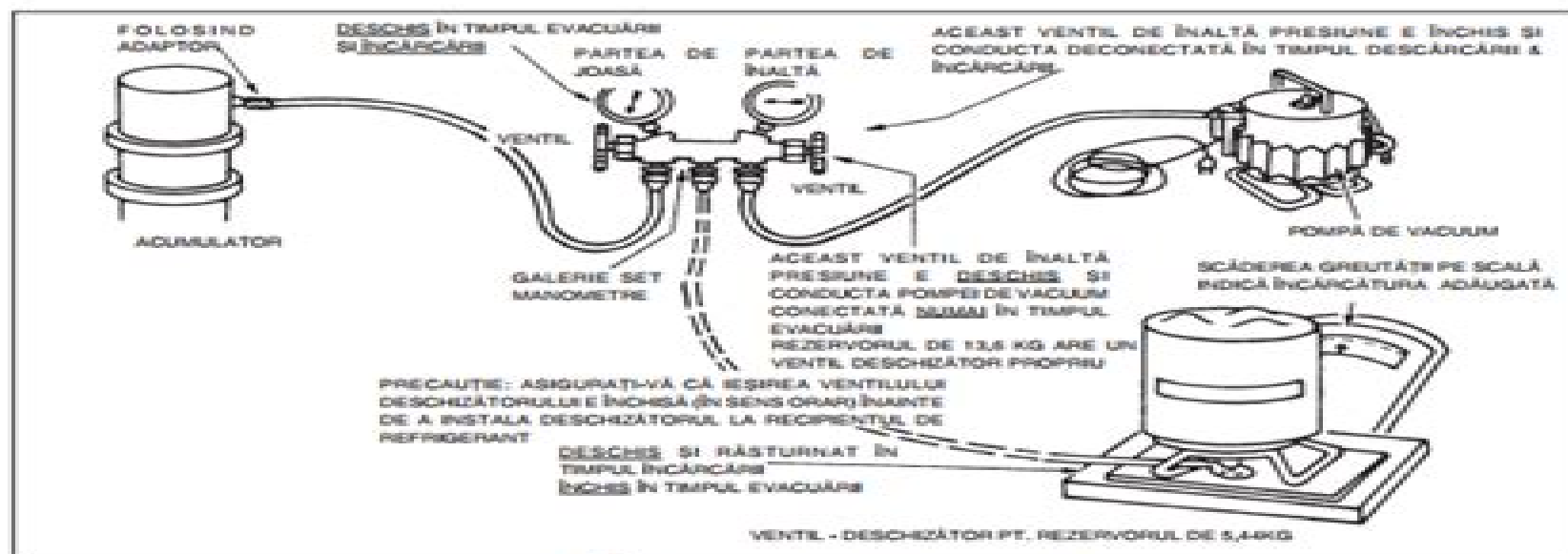
Fig. 14 Încărcarea sistemului cu rezervorul
