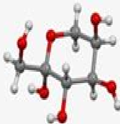
FRUCTOSE
