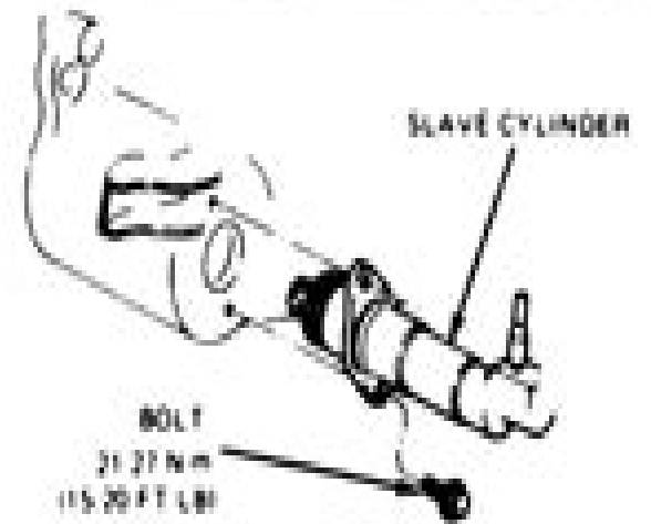
VIEW Y
