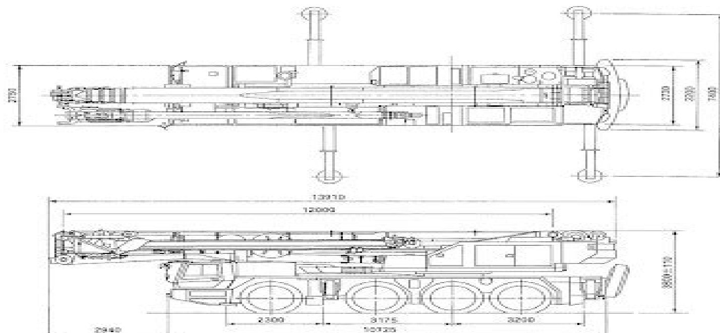
SA 1000 Min. Path Width for Square Turn
