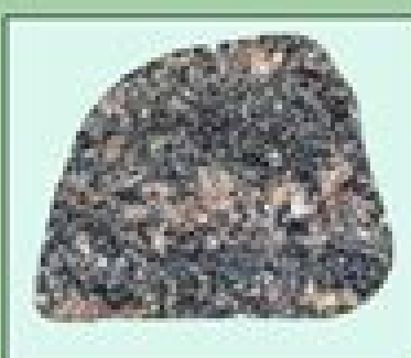
Migmatite
